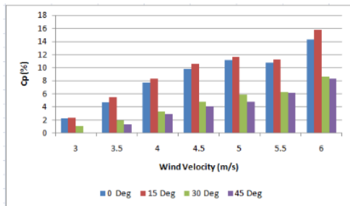
Gambar 5. Variasi Cp terhadap kecepatan angin
