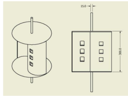
Gambar 2. Model Turbin Angin yang diteliti
