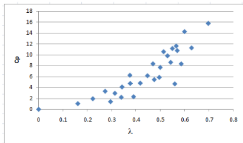
Gambar 6. Variasi Cp terhadap tip speed ratio
