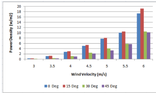
Gambar 4. Variasi Power density terhadap kecepatan angin
