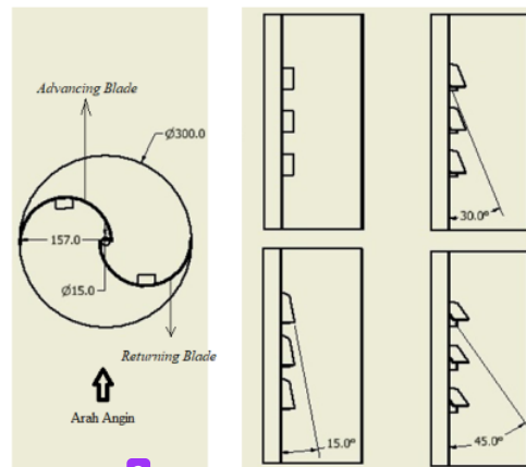
Gambar 3. Besar Sudut Bukaan Fix Drag Reducing
