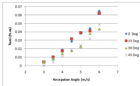
Gambar 9. Torsi model turbin angin terhadap kecepatan angin
